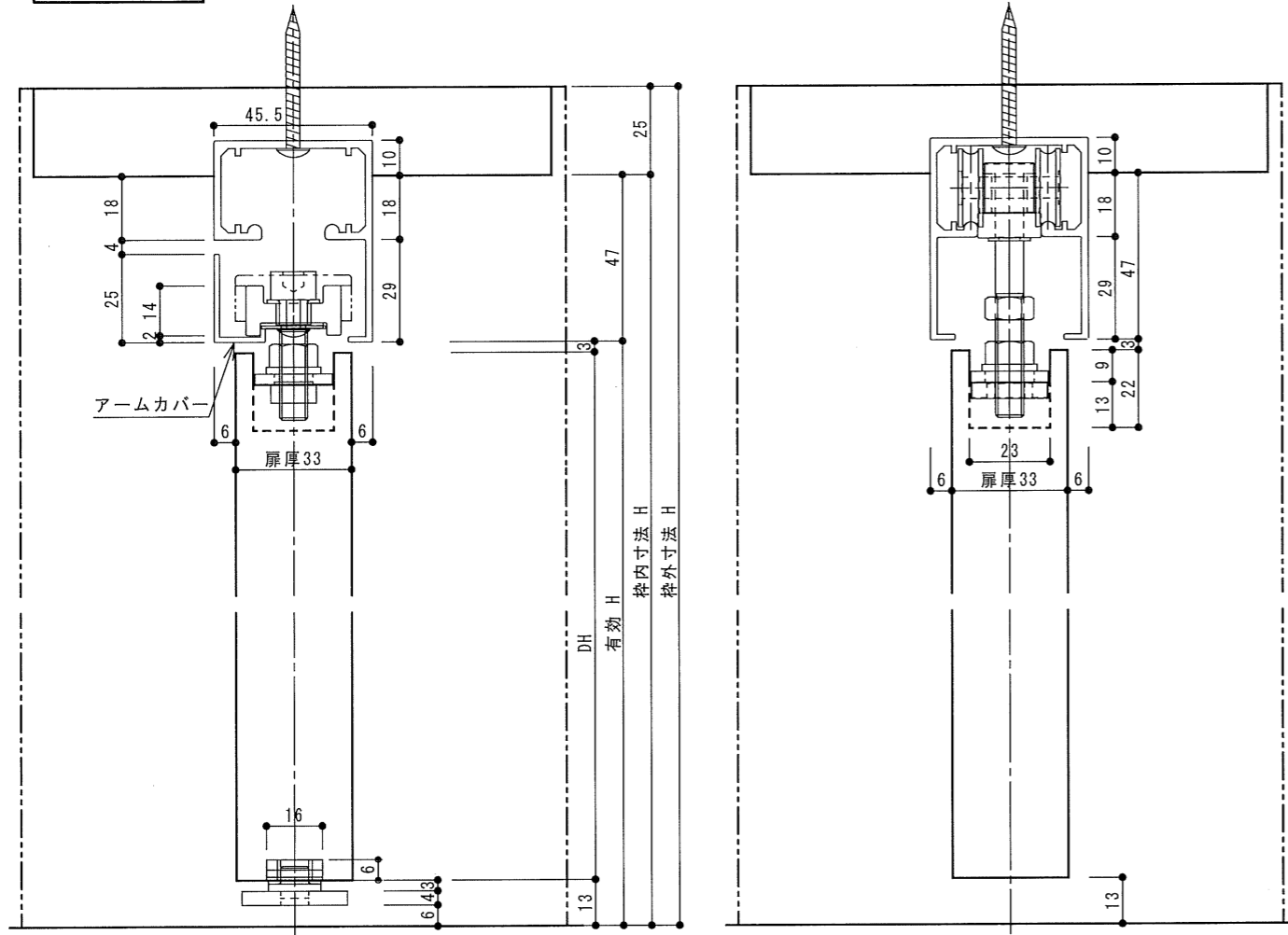
縦断面図
