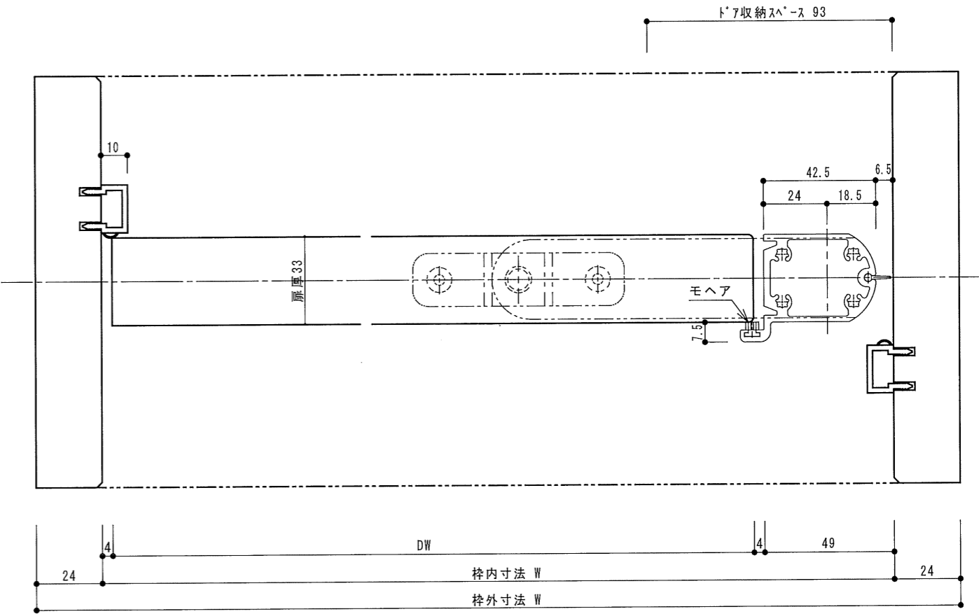
横断面図
