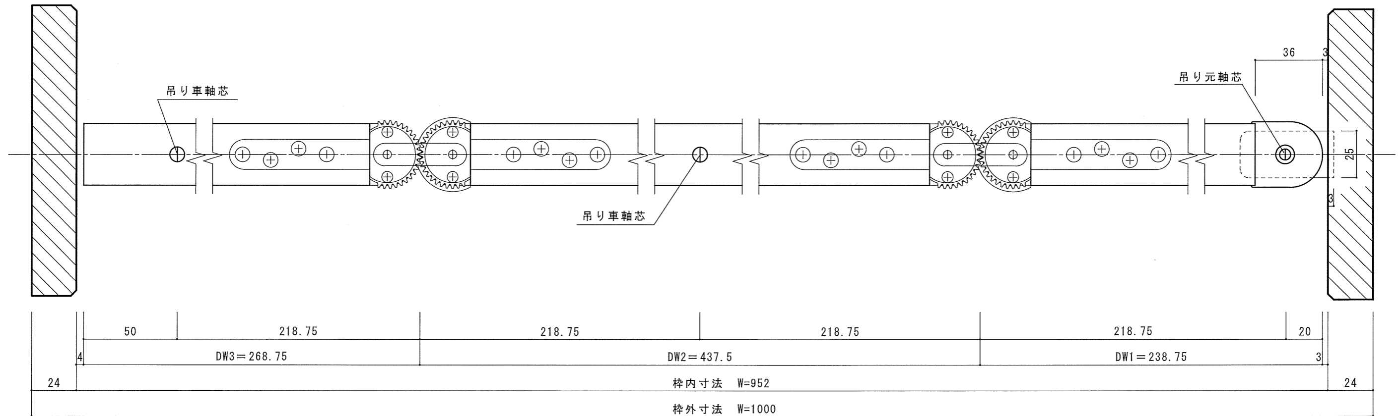
横断面図
