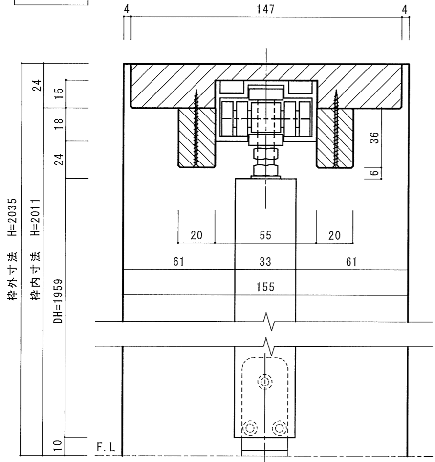
縦断面図
