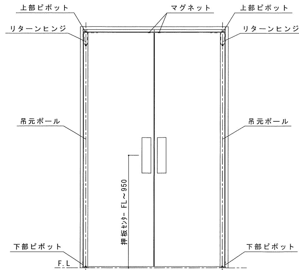
軌道図
