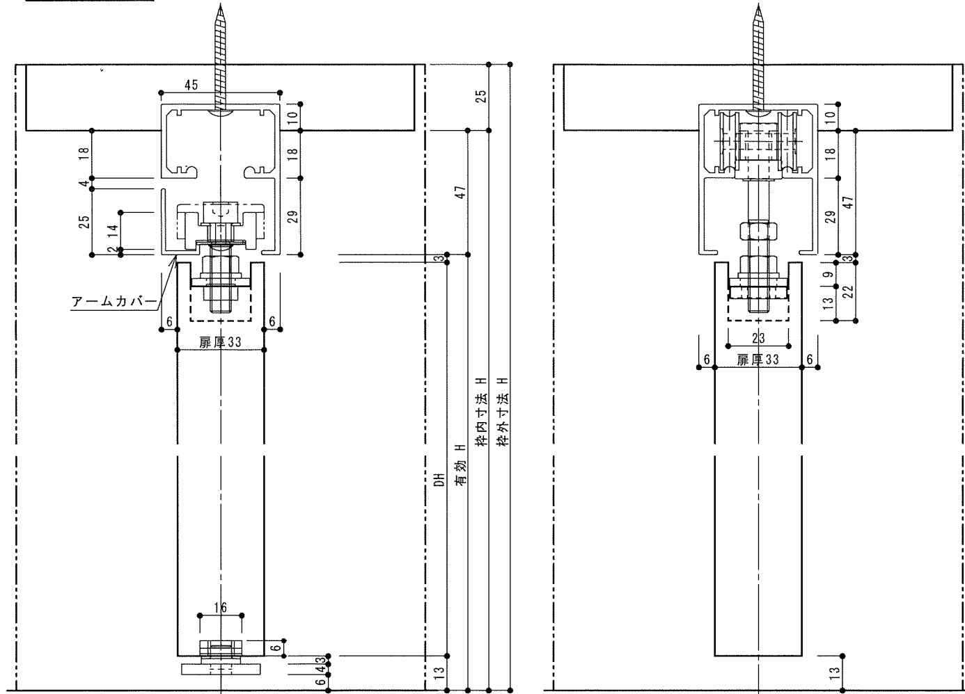
縦断面図
