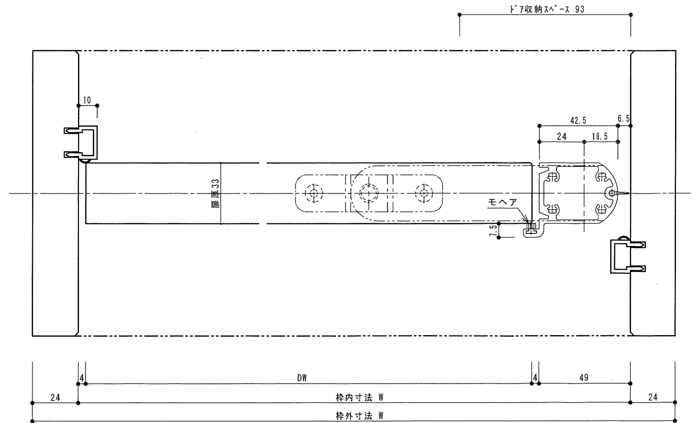
横断面図
